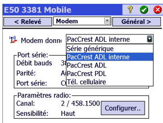
Onglet Modem de l'Epoch 50
